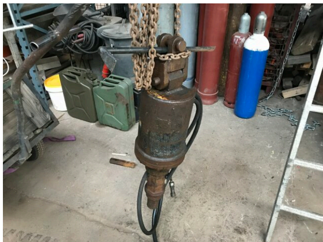
Kinshofer AS05 AS05 Antriebseinheit für Bohrschnecken
